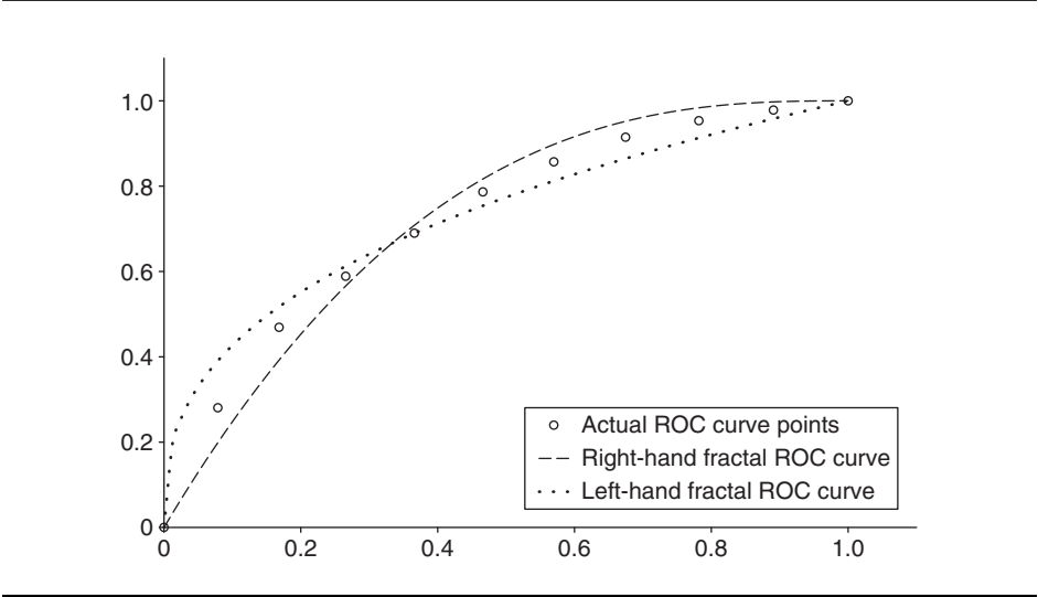
FIGURE 4 An empirical ROC curve from Řezáč and Řezáč (2011) versus right- and left-hand fractal ROC curves.
